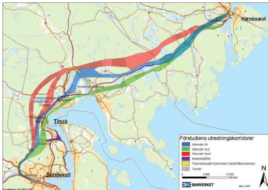
Figur 7 Utredningskorridorer för ny järnväg Sundsvall-Härnösand.
